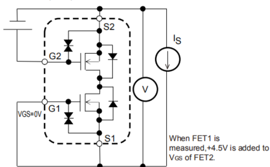
Test Circuit 7 VF(S-S)
