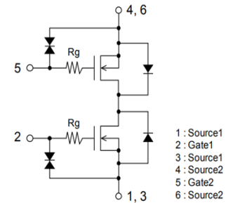
原理图 Schematic diagram
